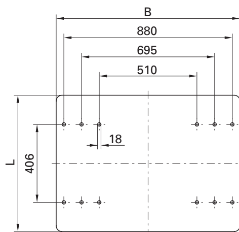
Схема отверстий DIN 74CB1 / ISO 3B42
